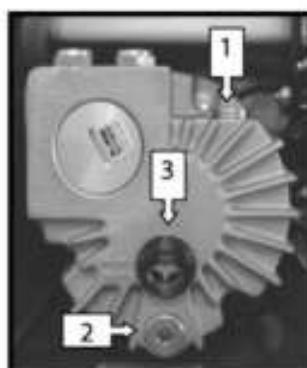
Вид сзади JUMBO PLUS (задняя панель снята)
