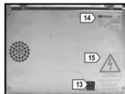
Вид сзади JUMBO 35 / 42
