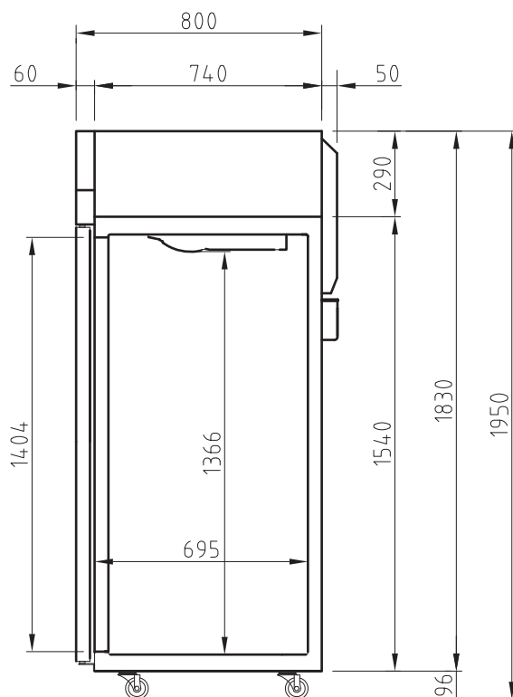
ВИД СБОКУ
