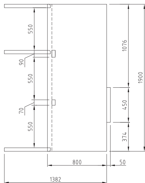
ВИД СВЕРХУ
