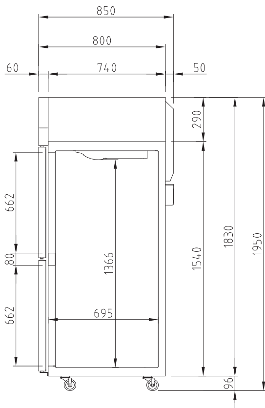
ВИД СБОКУ
