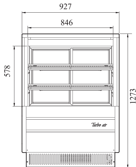
ВИД СПЕРЕДИ
