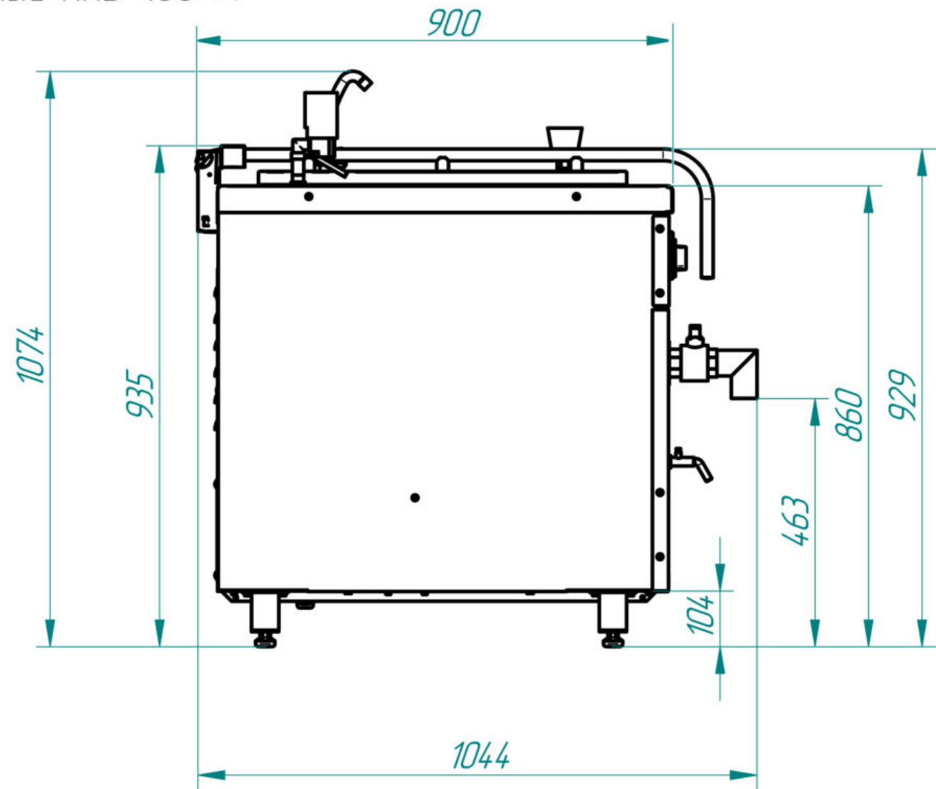
Котел пищеварочный КПЭ-100-М
