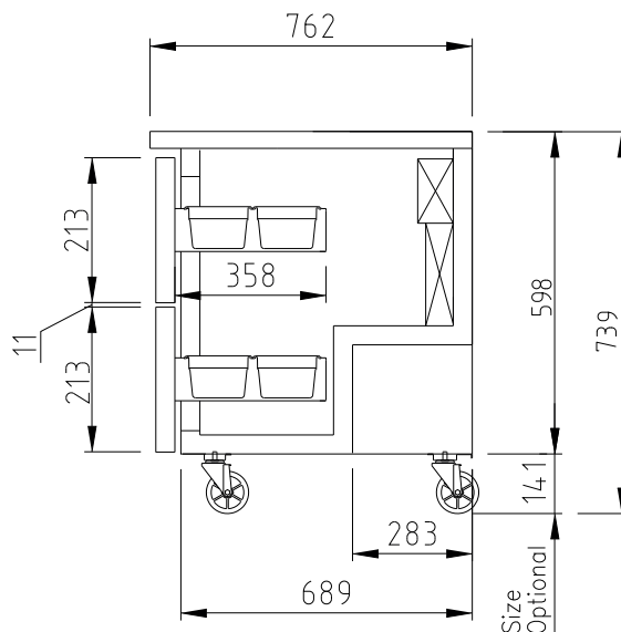
ВИД СБОКУ
