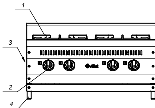
Рис. 2. Плита ПГК-47Н-П-А
