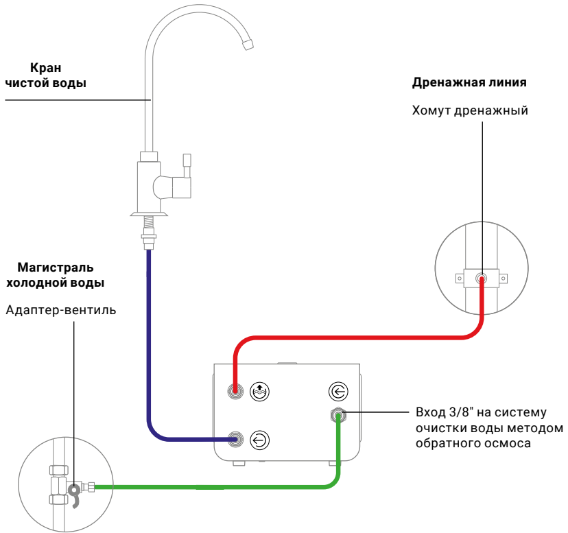
Рис. 2. Схема подключения системы Гейзер VIVO.
