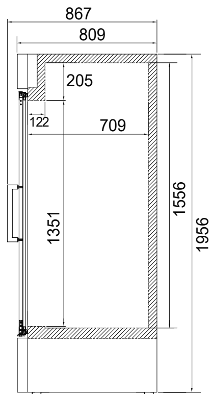
ВИД СБОКУ
