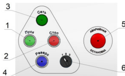
Рис. 2 Пульт управления
