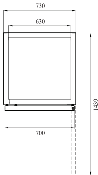
ВИД СВЕРХУ
