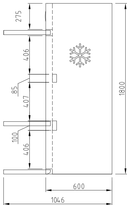
ВИД СВЕРХУ
