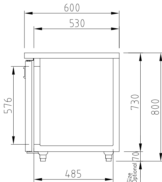
ВИД СБОКУ
