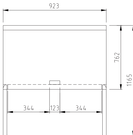
ВИД СВЕРХУ
