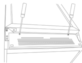
12. Das Bodenpaneel wieder montieren.
