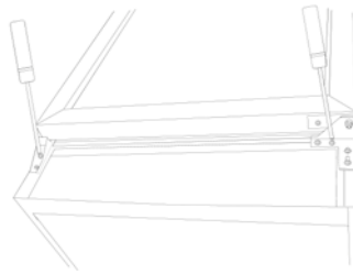
2. Démonter la charnière au fond et la ferrure de support.
