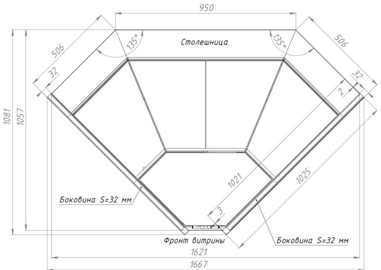
Витрина CALYPSO SLIM 3Y 90
