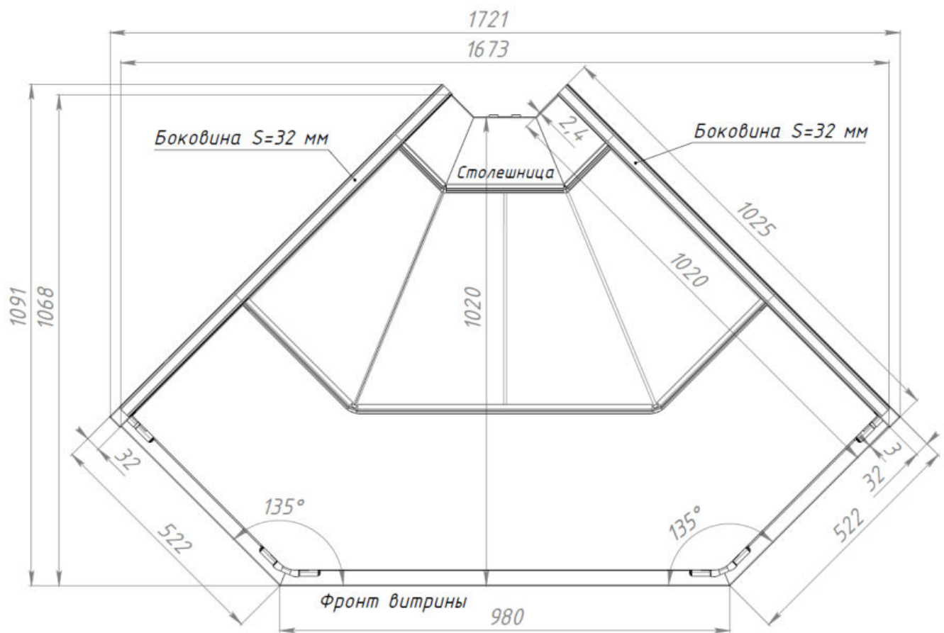
Витрина CALYPSO SLIM OY 90
