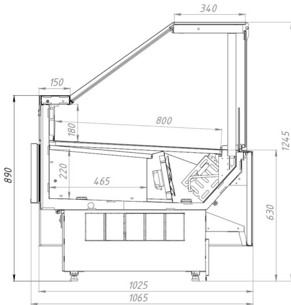
Витрина CALYPSO SLIM вентилируемая
