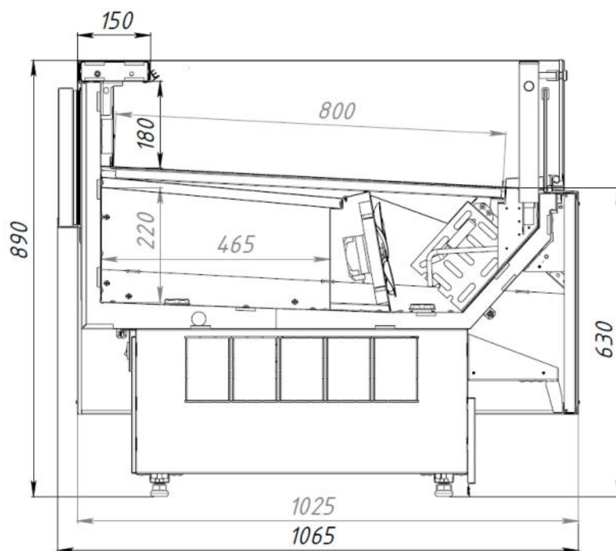
Витрина CALYPSO SLIM SELF вентилируемая
