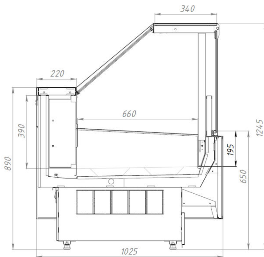
Витрина CALYPSO SLIM HT
