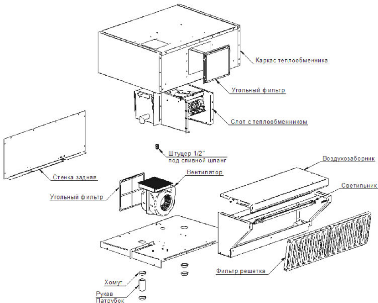
Рис 3 - Состав зонта
