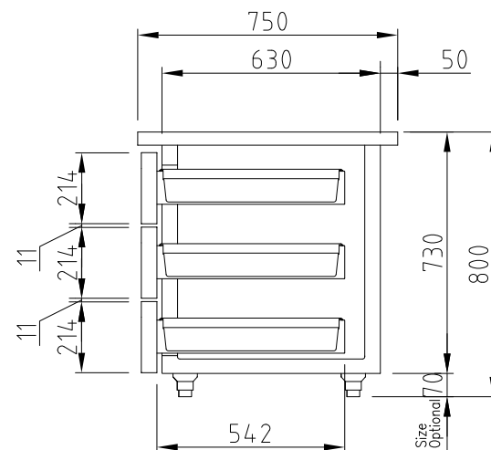
ВИД СБОКУ
