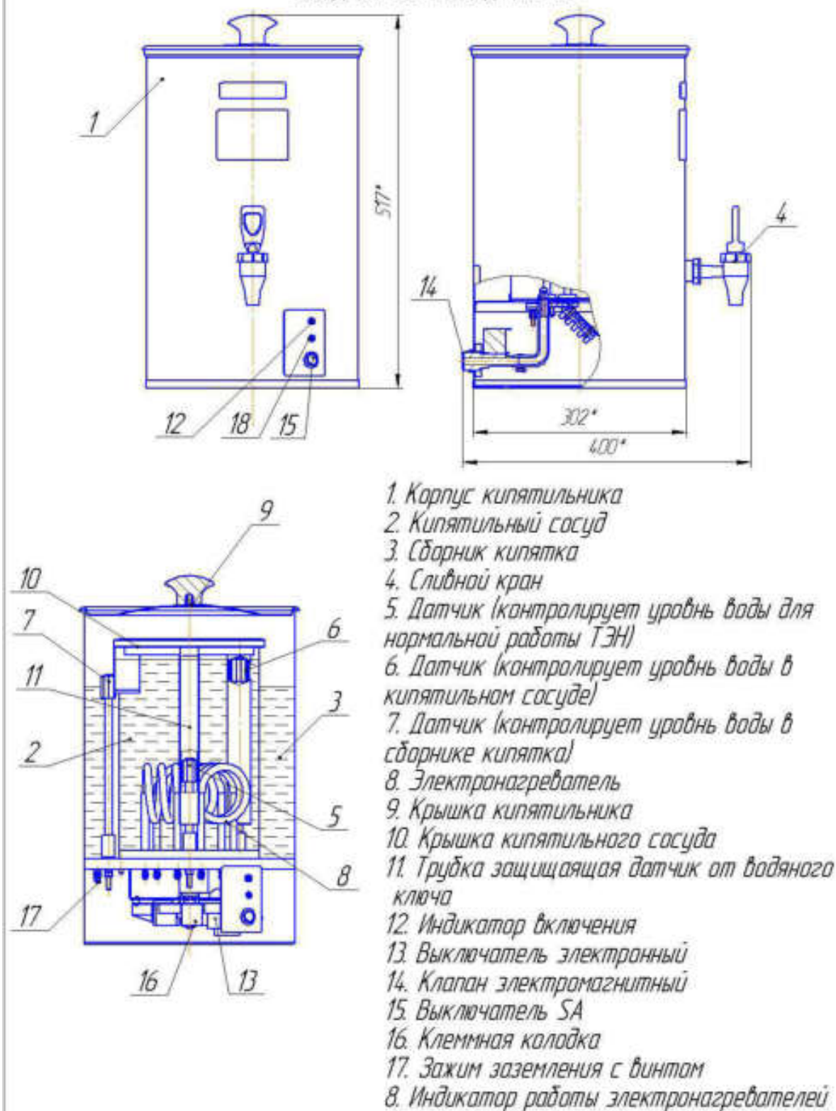
Общий вид кипяtilьников электрических непрерывного действия КЭНД-50-03 и КЭНД-100-03
