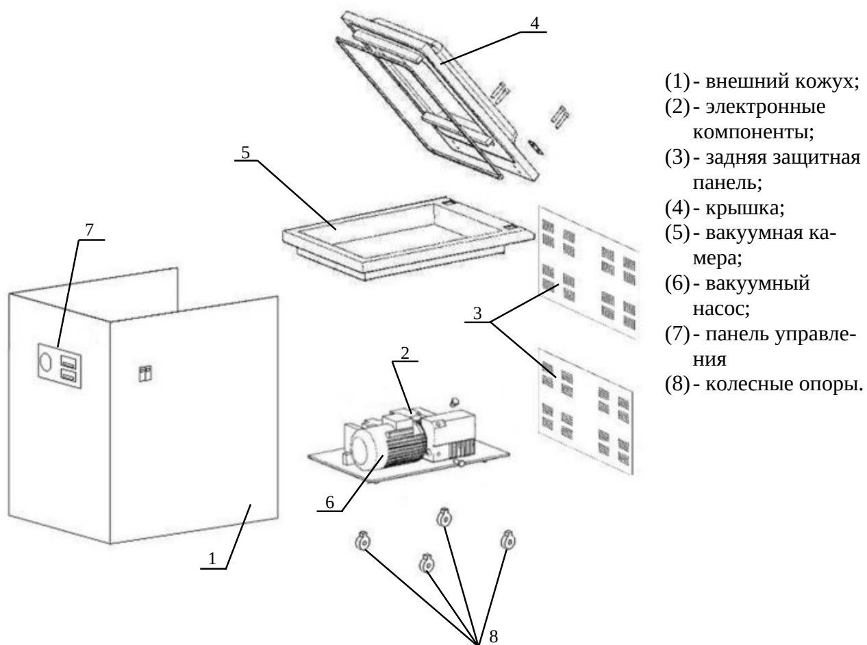
Рисунок 4.4 – Покомпонентный вид справа
