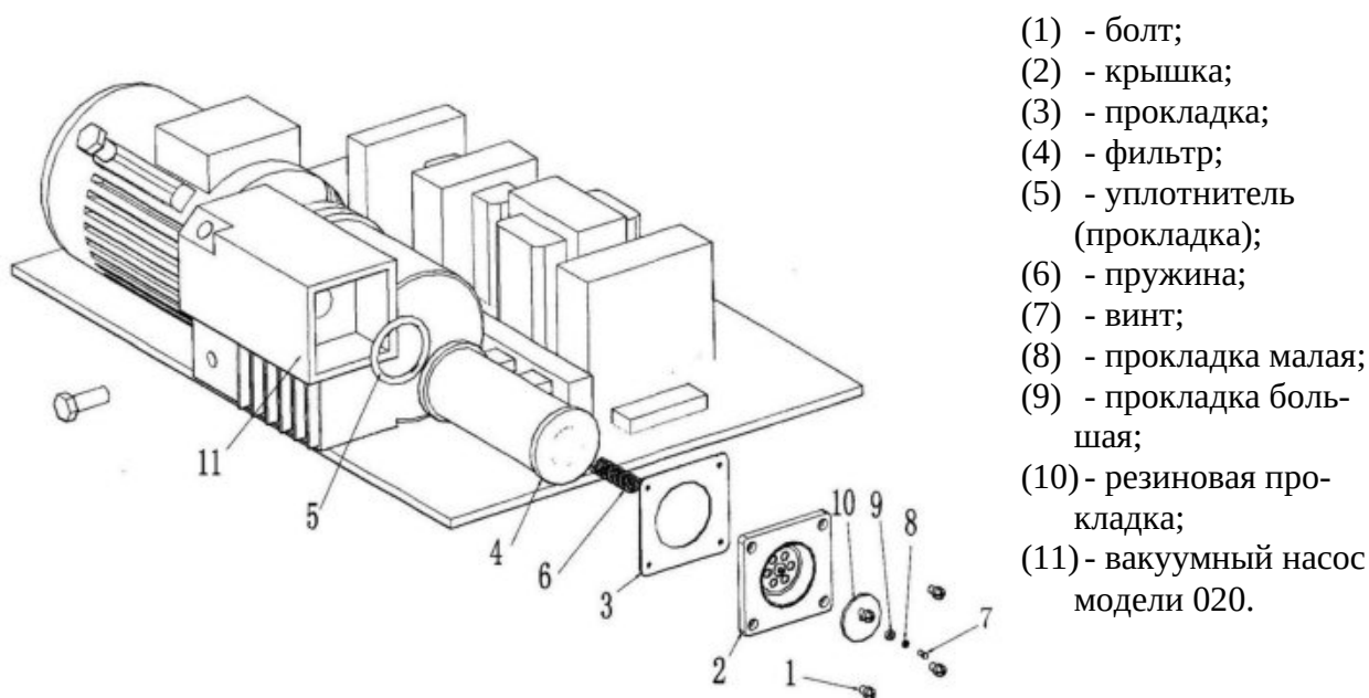
Рисунок 7.3 - Схема элементов вакуумного насоса модели 020
