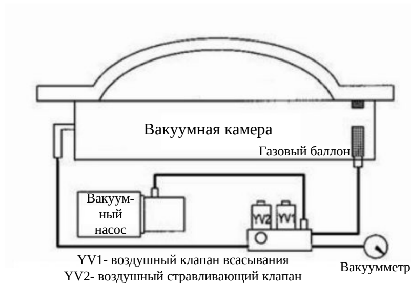
Схема вакуумного упаковщика с производительностью вакуумного насоса 10 м 3
