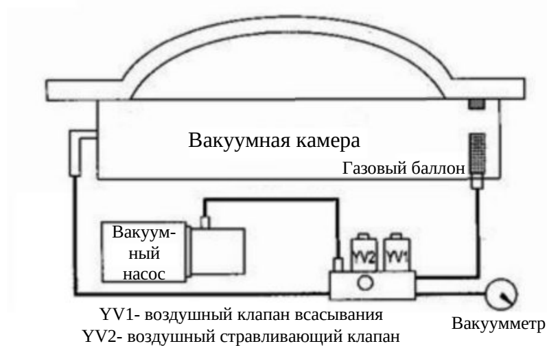
Схема вакуумного упаковщика с производительностью вакуумного насоса более 20 м 3
