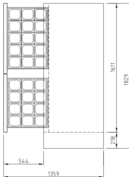
ВИД СВЕРХУ
