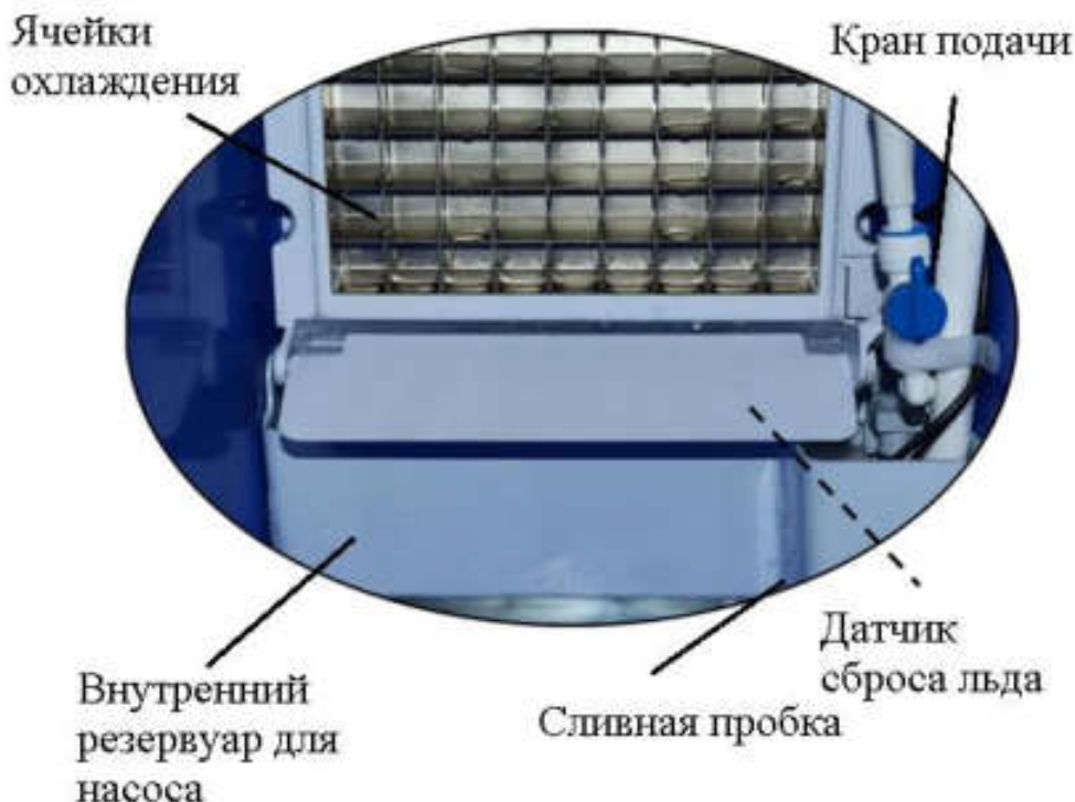
Рис. 3 Внутренности льдогенератора
