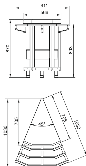
МП-45KM
