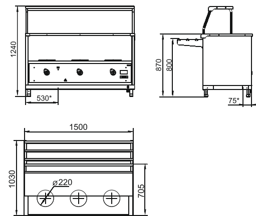
ПМЭС-70КМ-01
