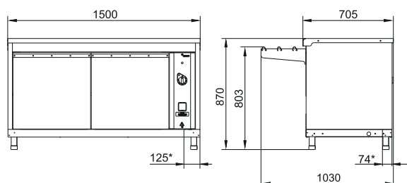
ПВТ-70КМ-02
