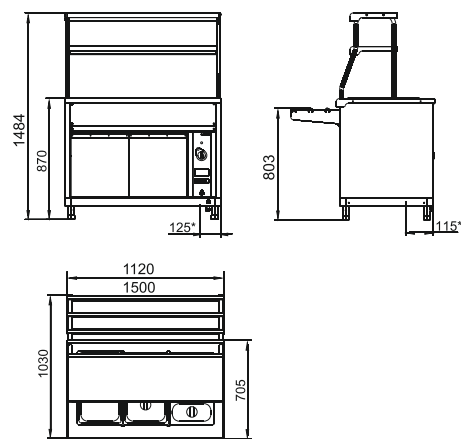
ПМЭС-70КМ-60, ПМЭС-70КМ-80
