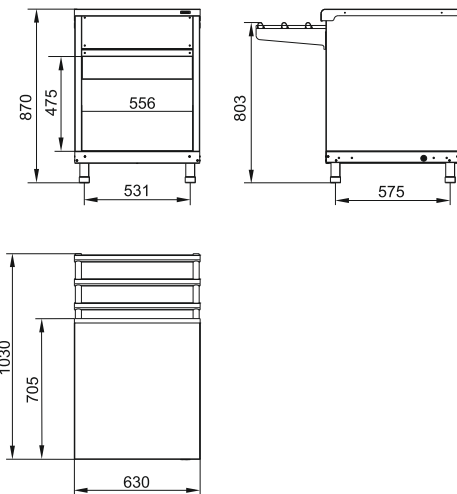
МН-70KM
