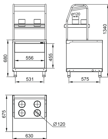
ПСПХ-70КМ
