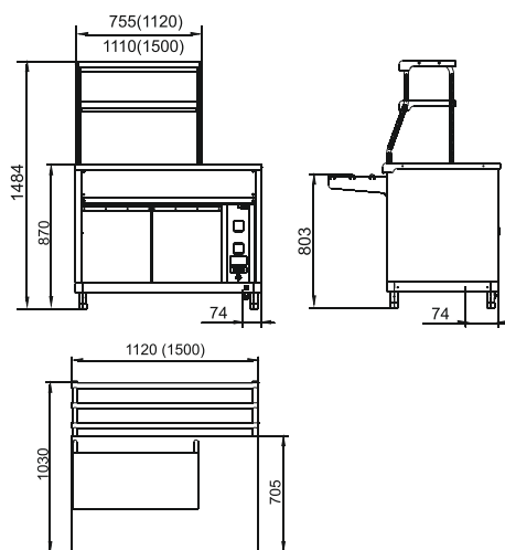
ПГН-70KM, ПГН-70KM-01
