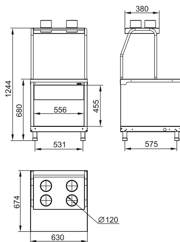
ПСП-70КМ
