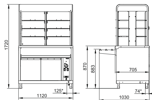
ПВТ-70КМ
