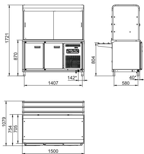
ПВВ(Н)-70КМ-С-01-ОК
