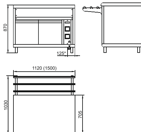
ПГН-70КМ-02, ПГН-70КМ-03
