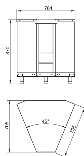
МП-45KM-01
