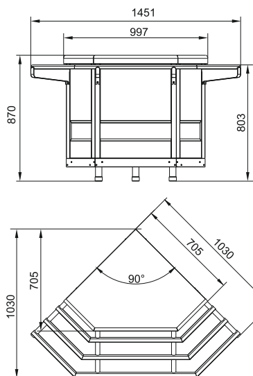
МП-90KM
