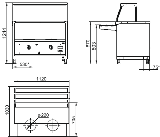
ПМЭС-70КМ-60, ПМЭС-70КМ-80
