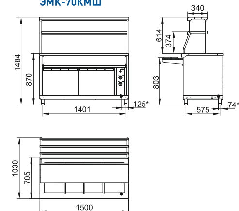
ЭМК-70КМШ
