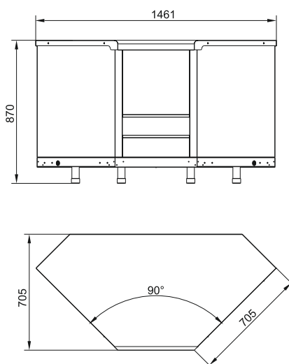
МП-90KM-01
