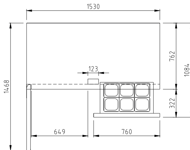
ВИД СВЕРХУ
