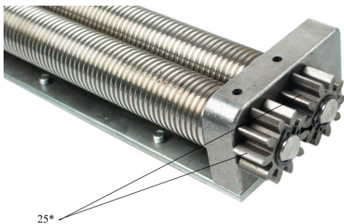
Рис3 Вид оборудования с правой стороны без защитного кожуха
