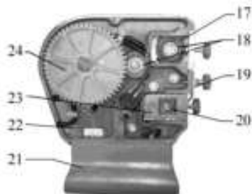
Рис 3: Вид внутри слева
