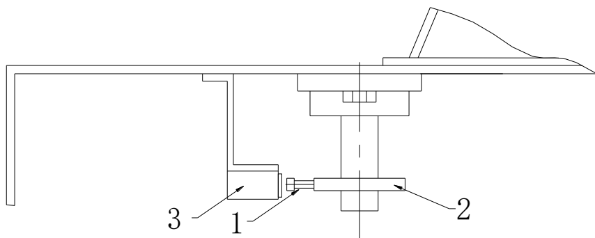
Рисунок 12 Регулирование процесса заполнения 1. Закручивающийся болт 2. пусковой полюс 3. датчик
