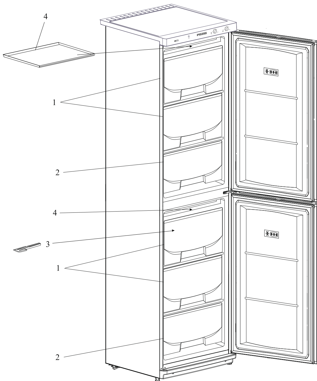
Рис. 1 Схема расположения отделений морозильника и его комплектующих
