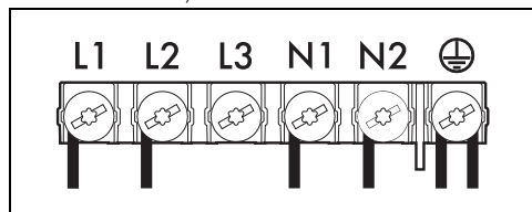
Шестижильный кабель 6 x 1,5 мм².
