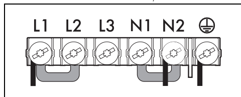
Трехжильный кабель 3 x 6 мм².
