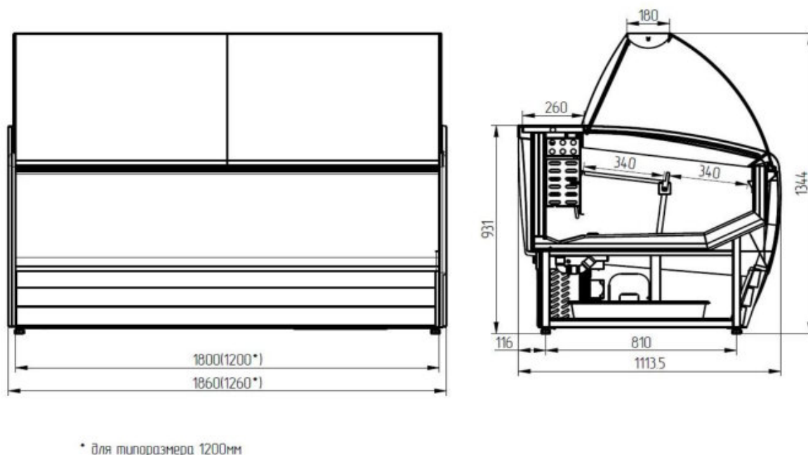
Рис. 1. Схема витрины «ВИЛИЯ ICE» ВН
