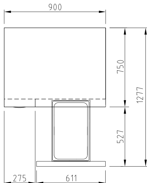
ВИД СВЕРХУ
