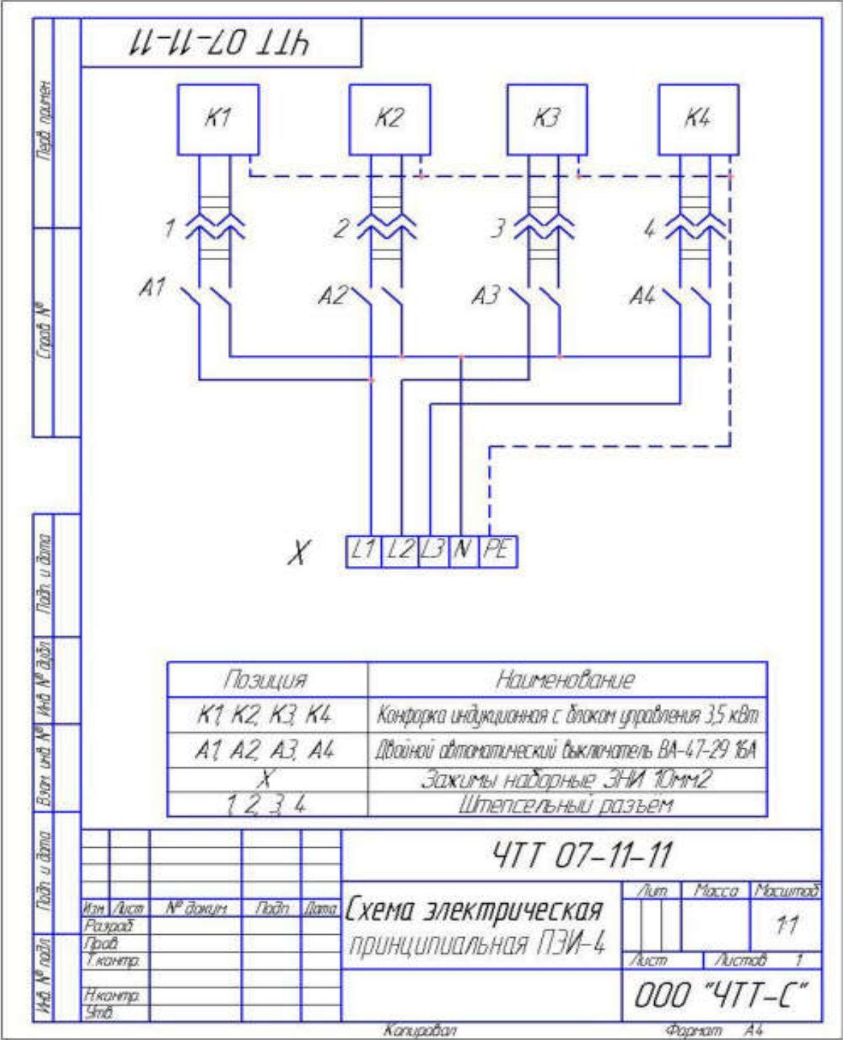
Схема электрическая принципиальная ПЭИ-4.
