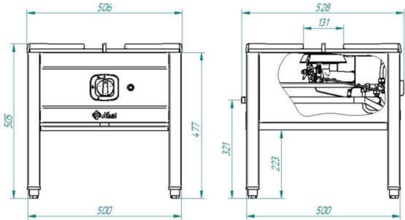
Габаритные размеры газовой плиты ПГК-15П-II-A
