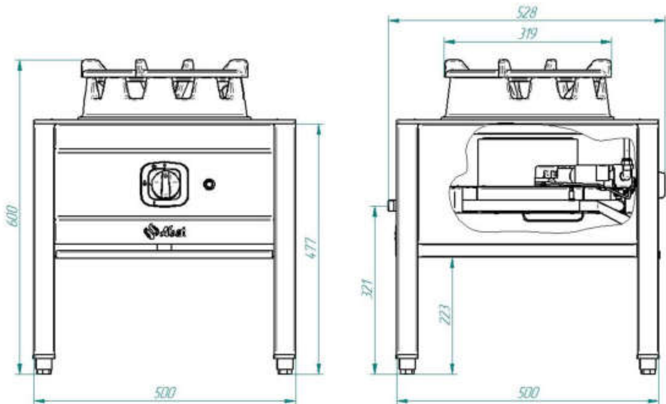
Габаритные размеры газовой плиты ПГК-15П-ВОК-II-A
