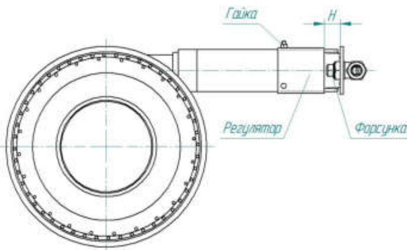
Рис.5 Горелка ВОК
