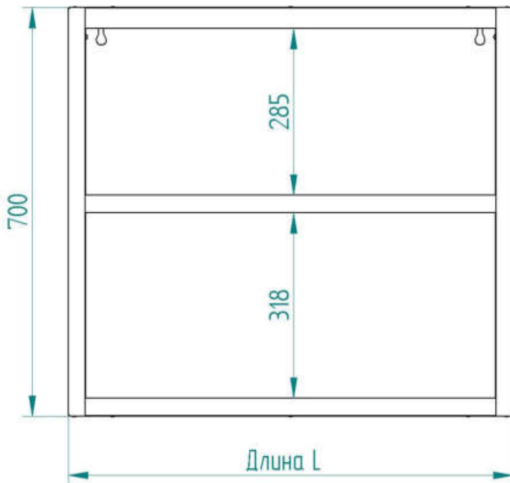
Рис. 3 Полка ПНО (вид спереди)
