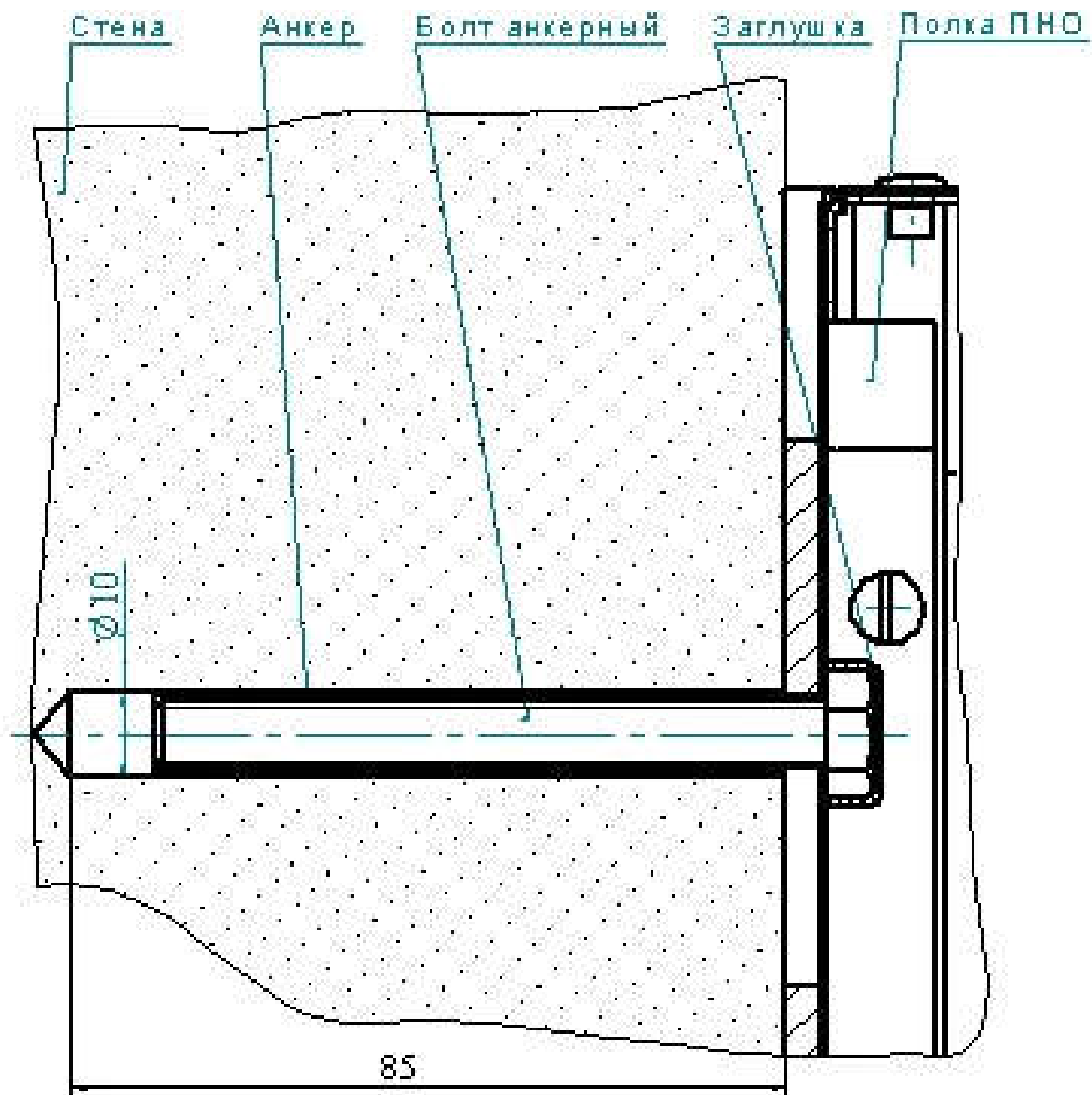
Рис.1 Пример крепления полки ПНО
