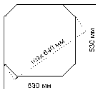
Размеры противня 530х530мм
