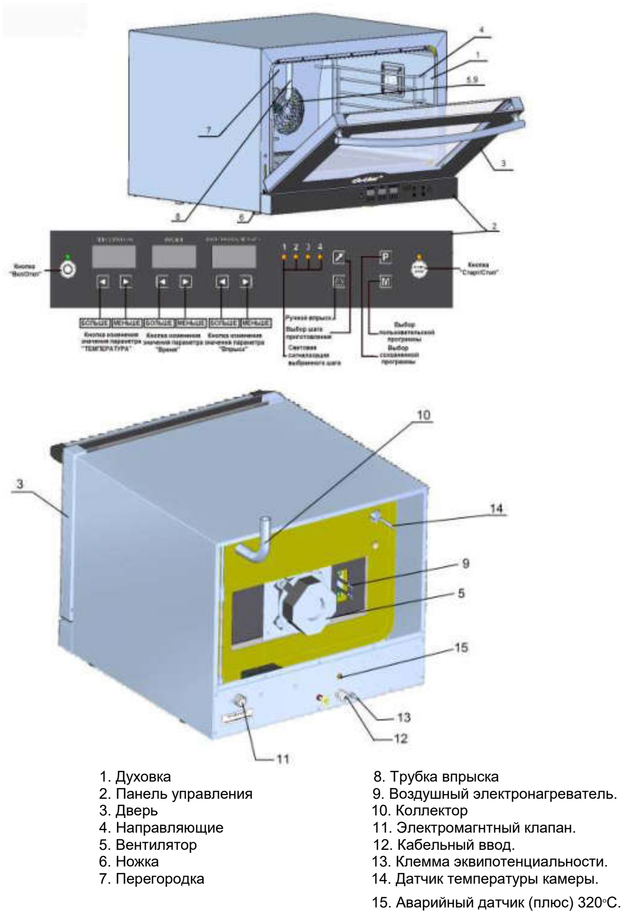
Рис. 1.2 Общий вид печи КПП-4П, КПП-4ПЭ и КПП-4-1/2П
