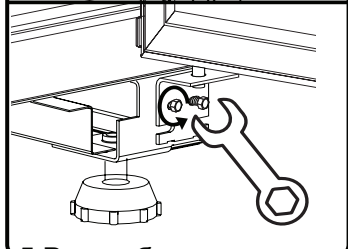
5. Расслабьте крепление у верхней и нижней петли.
