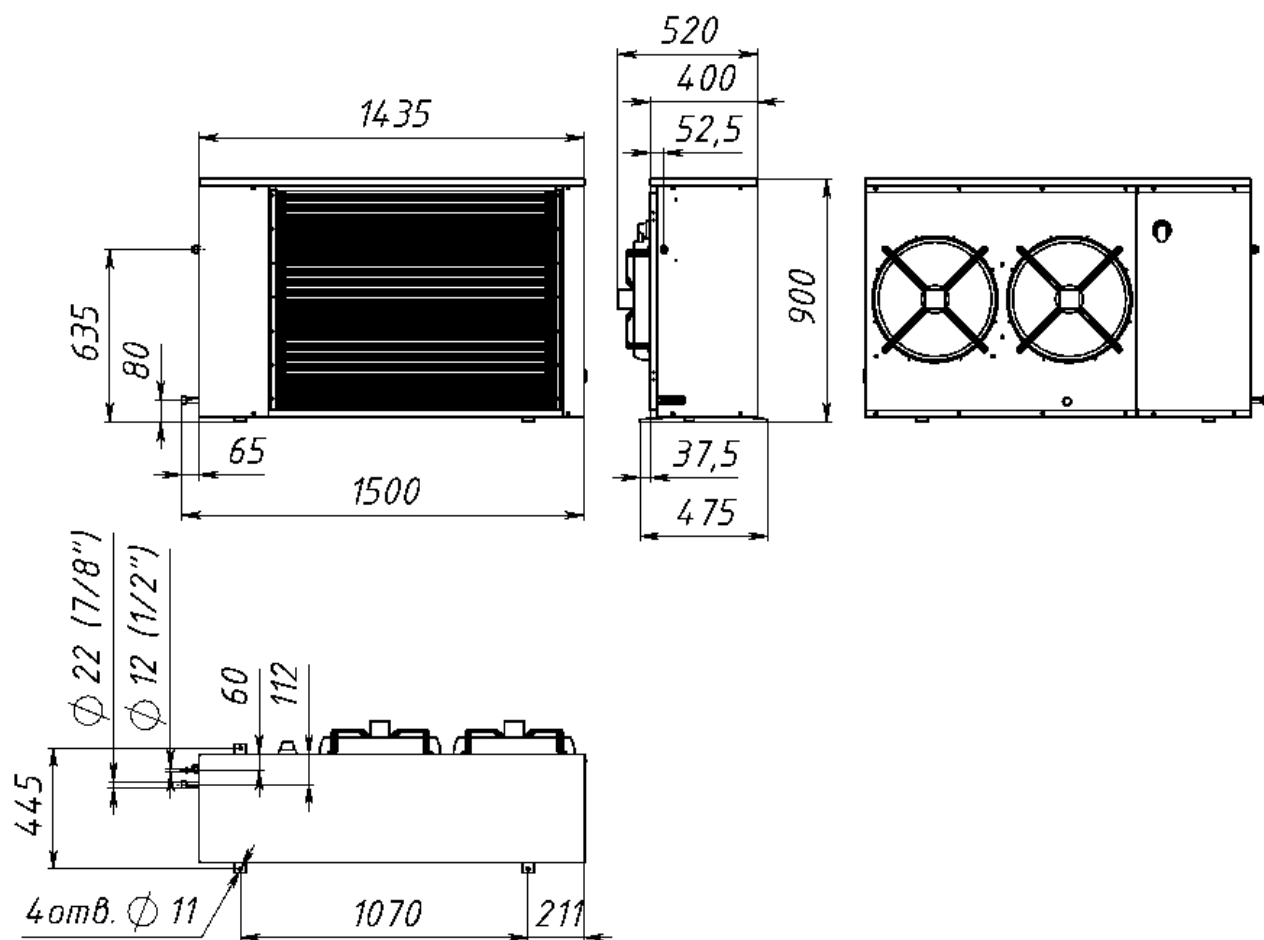
Общий вид агрегатов ZB45, ZB48
