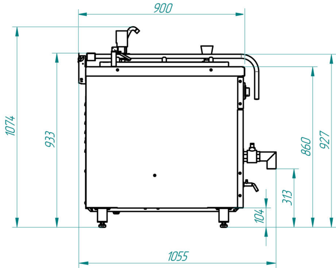
Котел пищеварочный КПЭ-160-М
