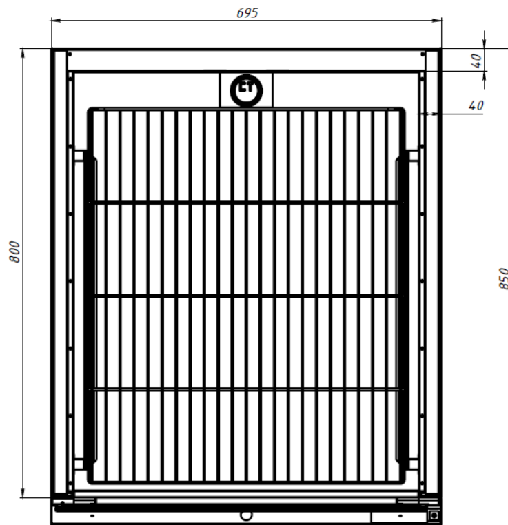
рисунок 3 – Сечение шкафа холодильного «Shkaff II 1400CT и 700CT»
