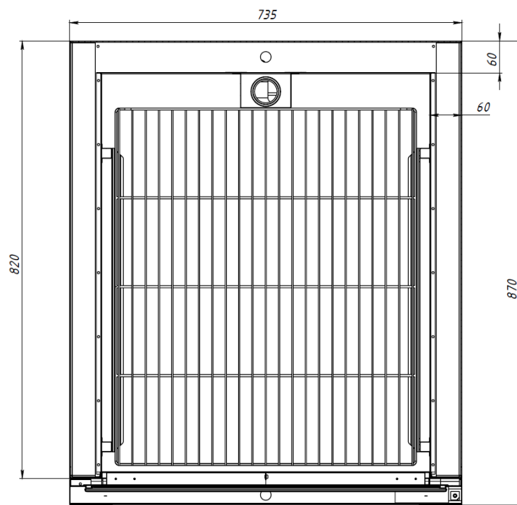
рисунок 2 – Сечение шкафа холодильного «Shkaff II 1400HT и 700HT»
