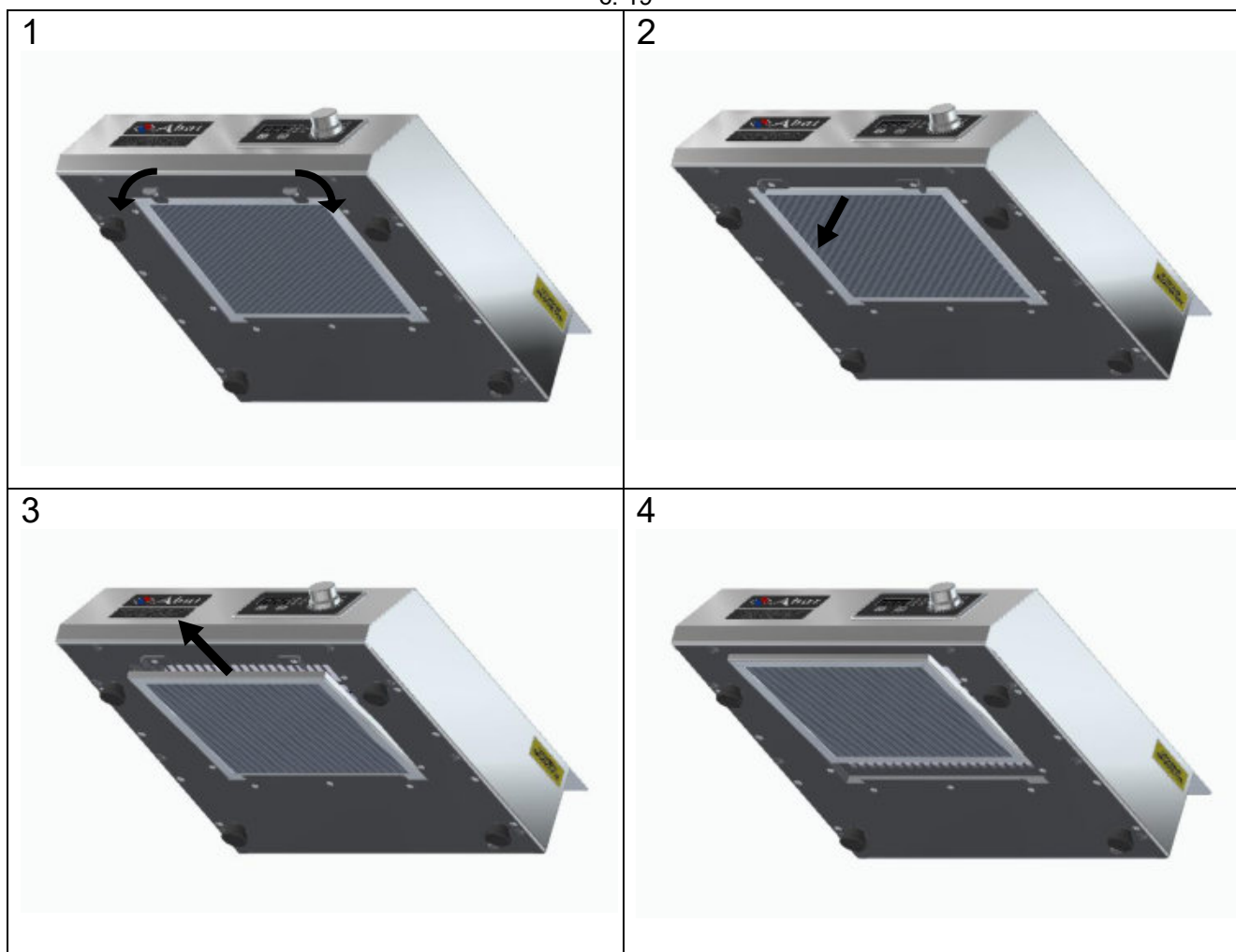
Рис. 4. Извлечение жировлавливающего фильтра
