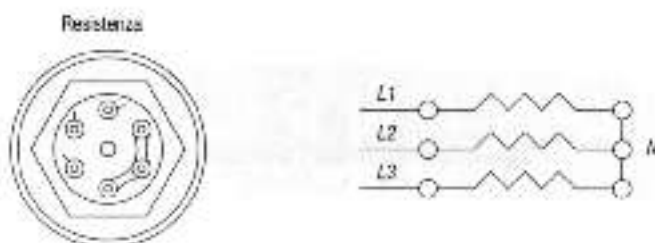
Variante alimentazione elettrica
