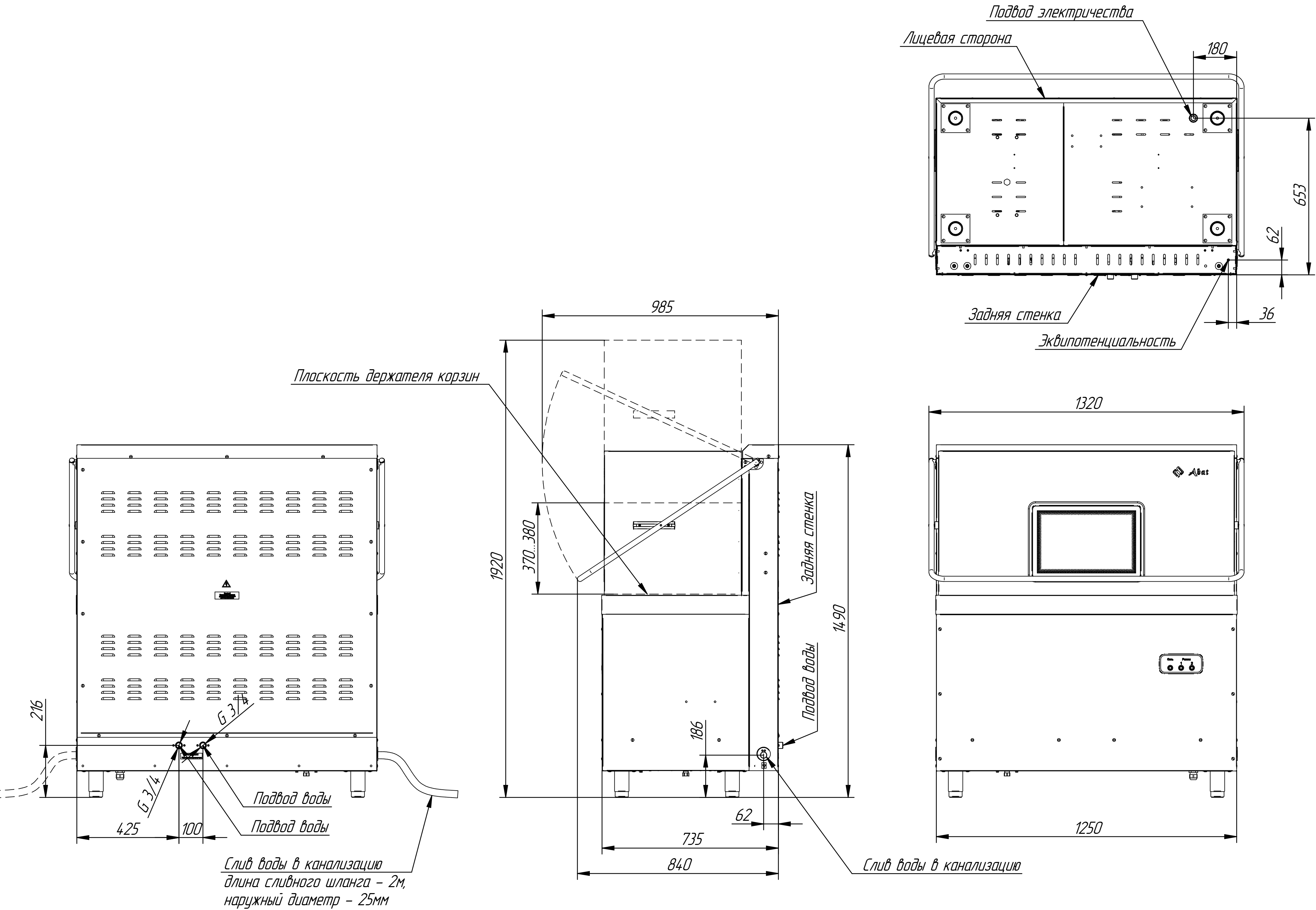
Схема подключения машины МПК-1400К
