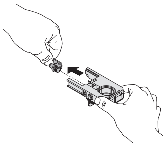
Промойте детали под струей воды. Убедитесь, что все отложения / остатки молока удалены. После мытья соберите детали в противоположном порядке.
