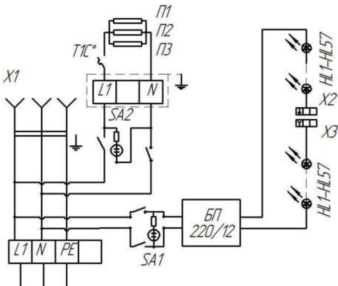
Мармит для вторых блюд RM23A Case. Схема электрическая принципиальная.
