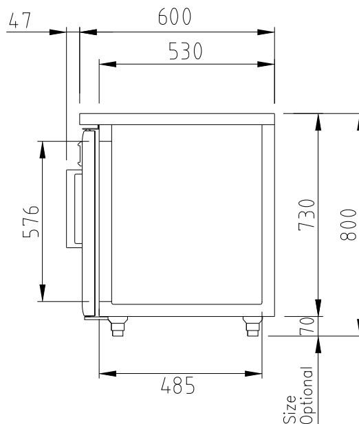
ВИД СБОКУ
