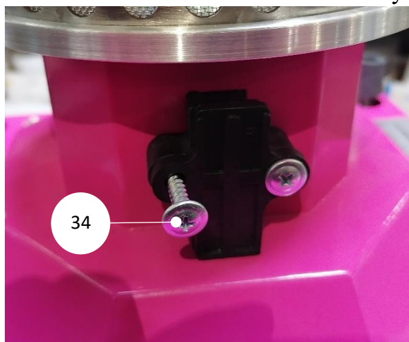
Рисунок 6 – Щеточный узел
