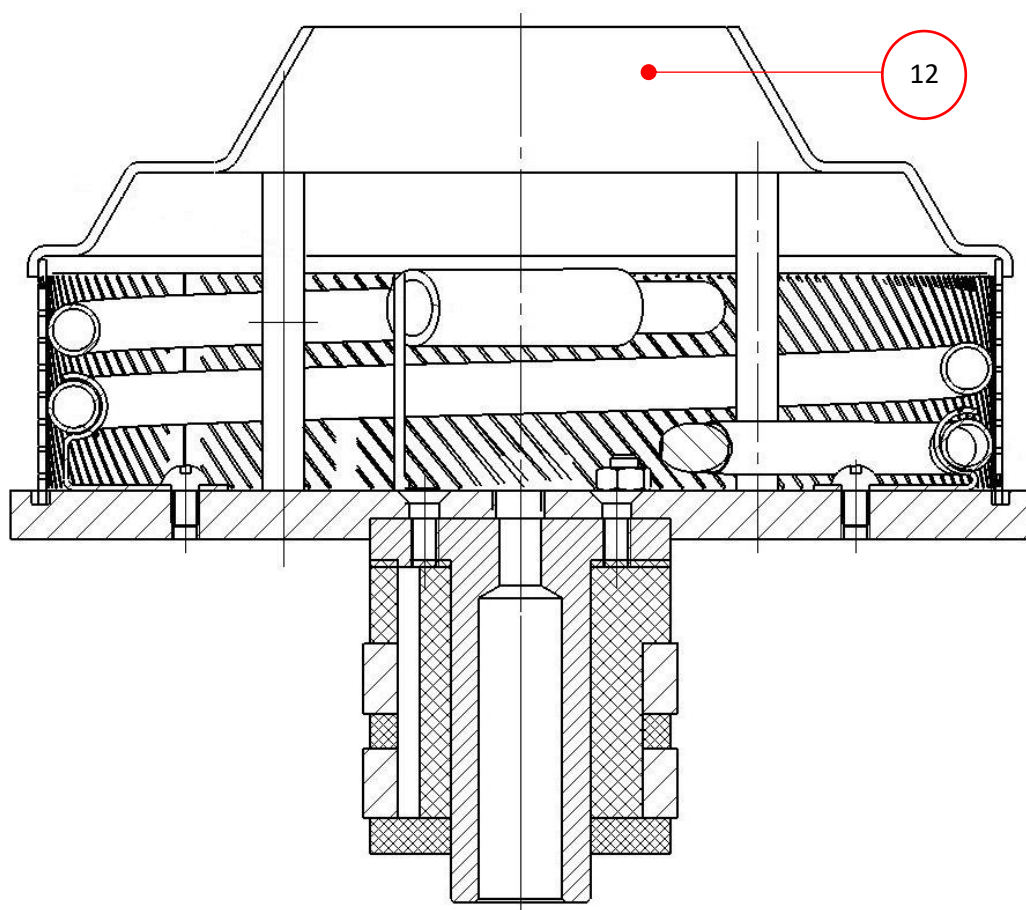
Рисунок 4 – Голова в сборе
