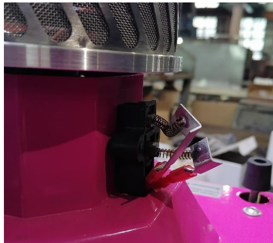
Рисунок 6 – Щеточный узел
