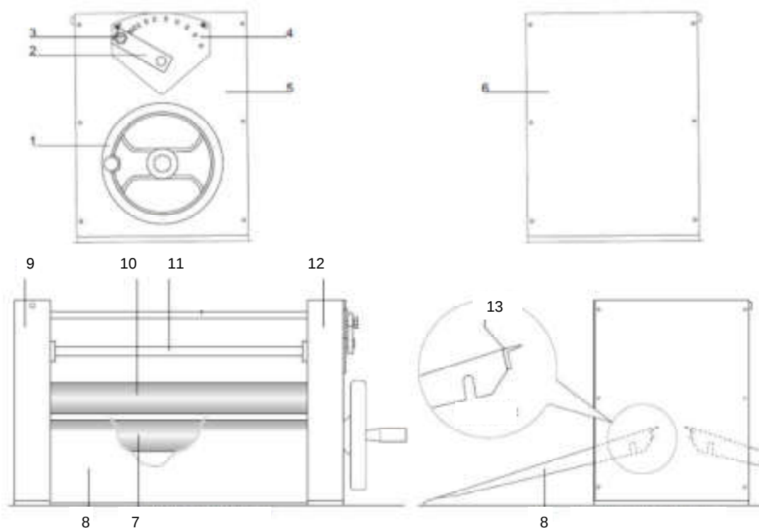
Рис.2 (компоненты машины)
