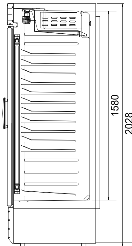
ВИД СБОКУ
