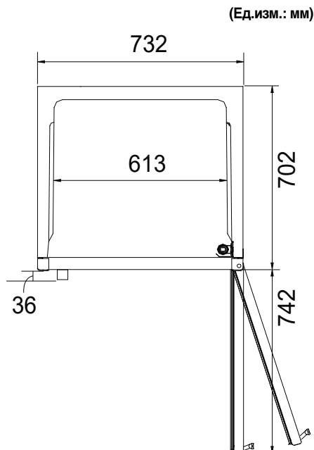
ВИД СВЕРХУ
