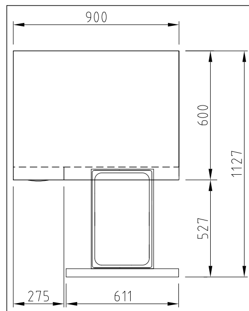
ВИД СВЕРХУ
