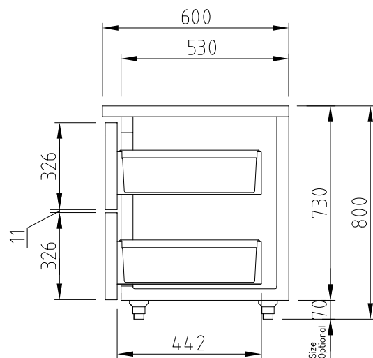
ВИД СБОКУ
