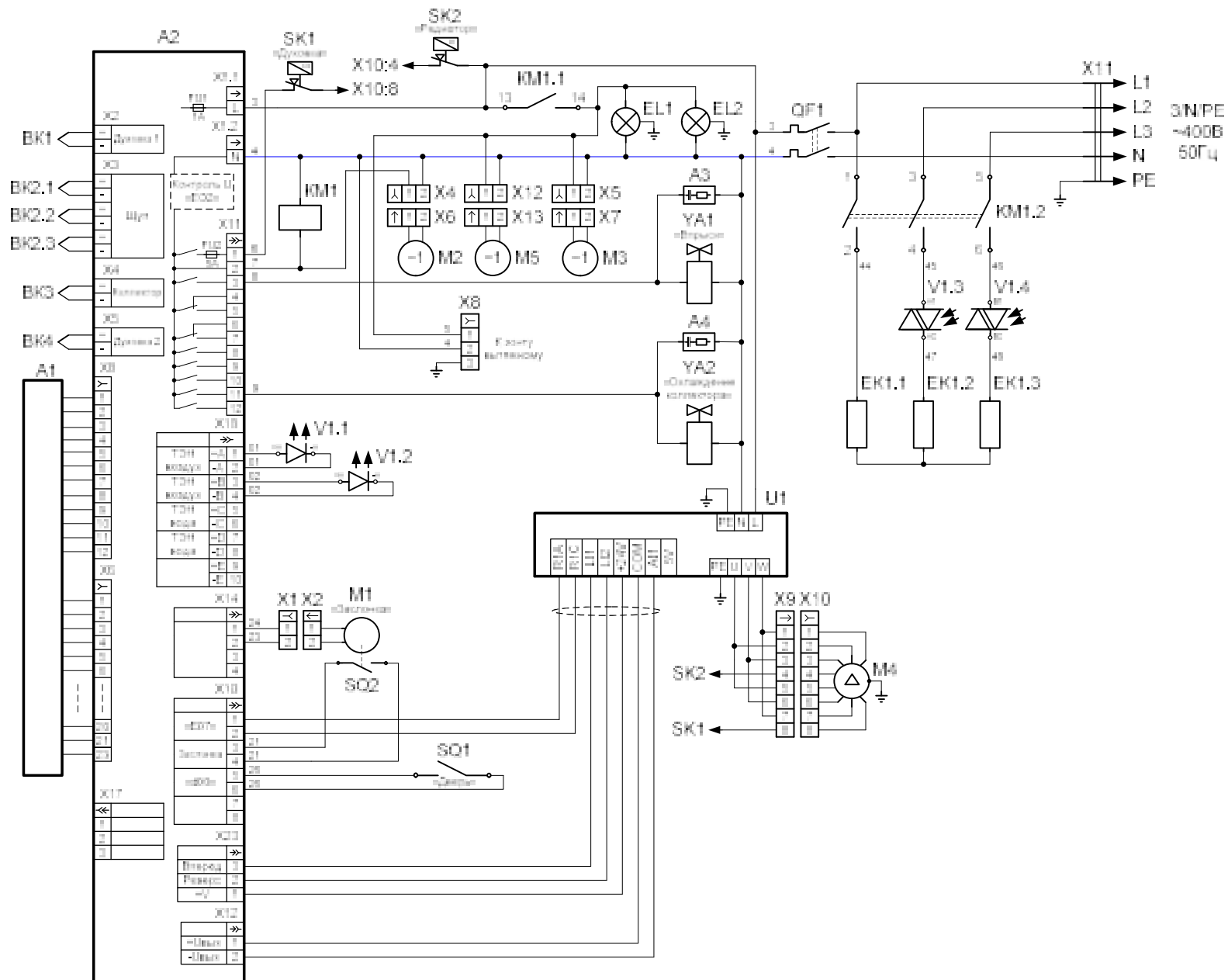
СХЕМА ЭЛЕКТРИЧЕСКАЯ ПРИНЦИПИАЛЬНАЯ ПКА6-1/1ВМ2 И ПКА10-1/1ВМ2
