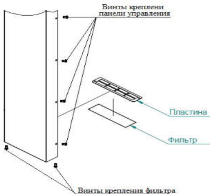
Рис. 13. Замена воздушного фильтра
